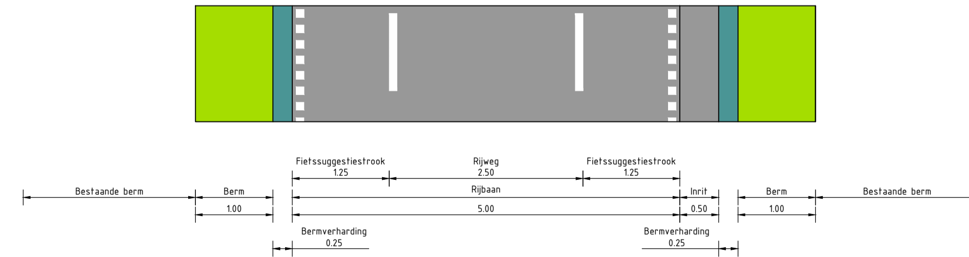
Principeprofiel Aanwassenweg Schaal 1:50
